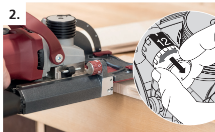
Fräsung in die Kante mit der 2 mm Aufsteckplatte (Frästiefe 12 mm)
