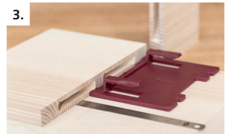
Fachboden als Anschlag mit Hilfe der Aufsteckplatte 2 mm versetzt ausrichten
